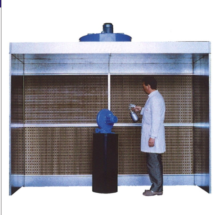
Abbildung: Ausführung NB mit Dach und Seitenwände um 1.000 mm verlängert
